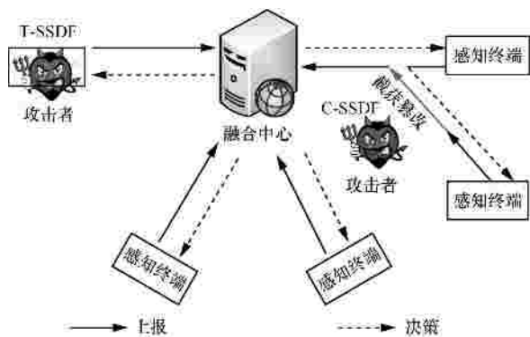
图 4 SSDF 攻击
