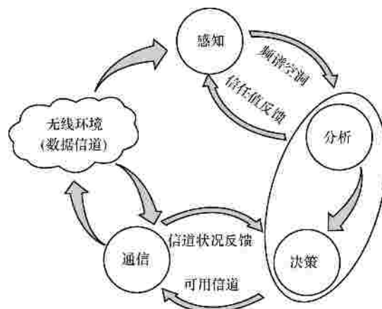
图1 认知环
