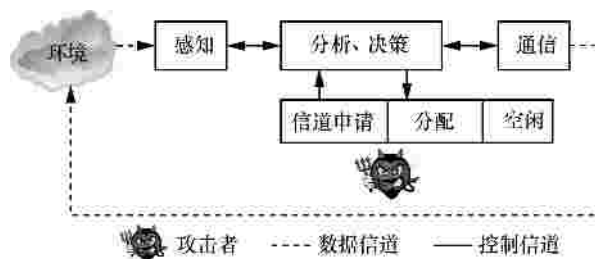
图 6 虚假申请
